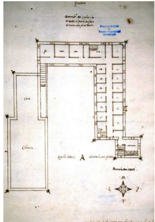
Obr. č. 28–29: Ideální půdorys přízemí (č. 28) a prvního patra (č. 29) kapucínského konventu (pro 14 členů) pro země se studenějším podnebím PAKÖS, Niederlassung Innsbruck, PANTP, sign. Fasc. 19, Libri tre nei quali si scuopre in quanti modi si puo edificare vn Monasterio (...)
