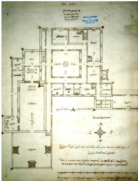
Obr. č. 28–29: Ideální půdorys přízemí (č. 28) a prvního patra (č. 29) kapucínského konventu (pro 14 členů) pro země se studenějším podnebím PAKÖS, Niederlassung Innsbruck, PANTP, sign. Fasc. 19, Libri tre nei quali si scuopre in quanti modi si puo edificare vn Monasterio (...)
