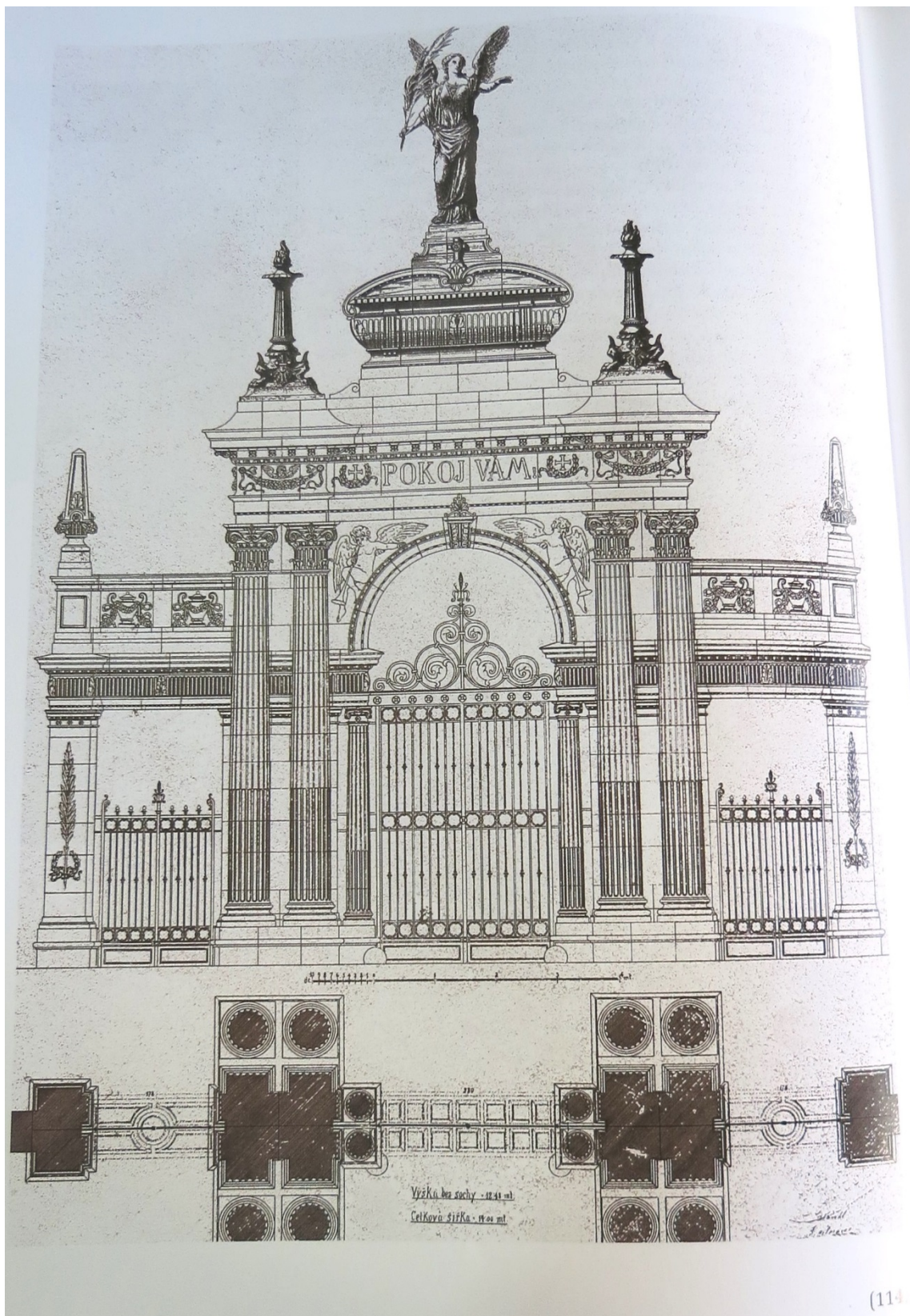
7. Bohuslav Moravec: plány portálu pro Nový hřbitov v Hořicích, 1891–1892
