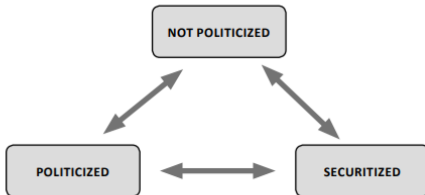
Obr. 1 – Schéma vztažnosti sekuritizace (Baysal, 2019, s. 6)
