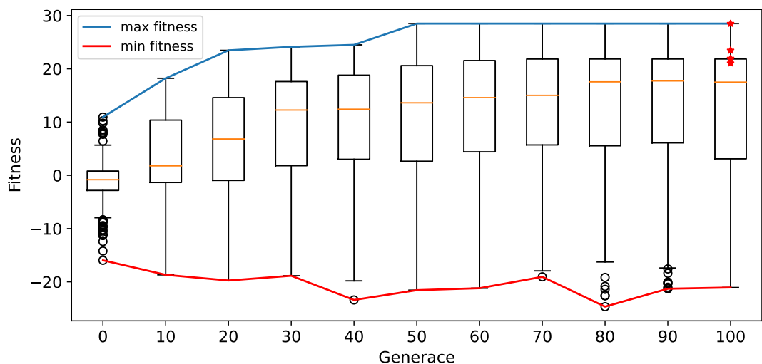
Obrázek 4.5: Vývoj fitness populace s pokročilým agentem TFSAgent a jednodušším robotem AntV3
