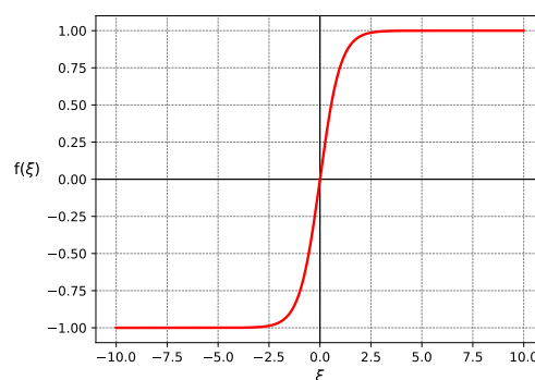
Obrázek 1.2: Funkce tanh
