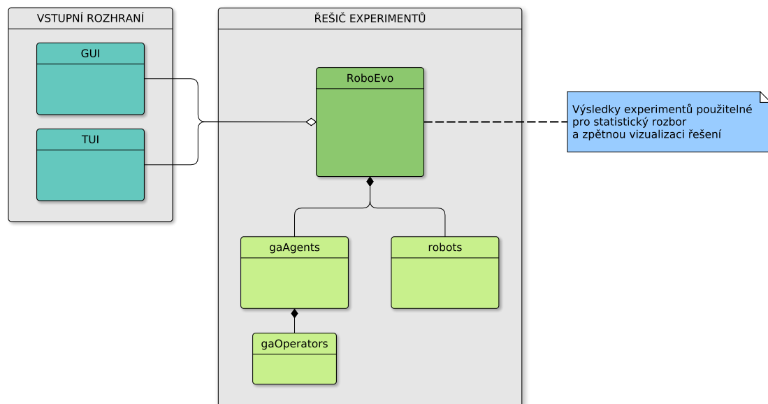
Obrázek 3.1: Struktura projektu
