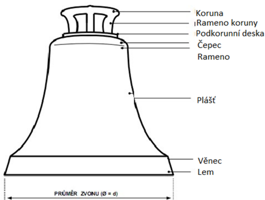
Obr. č. 13. Popis jednotlivých částí zvonu.
