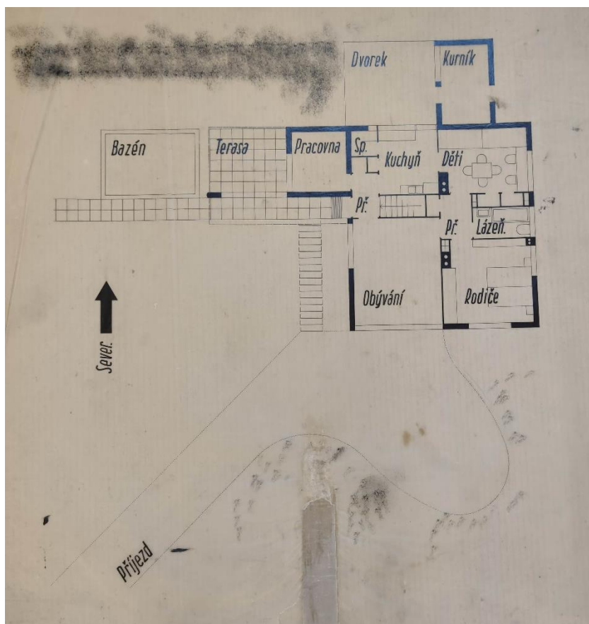
45. Lubomír a Čestmír Šlapetovy, Vila Josefa Kotoučka, Příbor-Klokočov, 1932–1933, půdorys vily s rekreační zahradou a příjezdovou cestou
