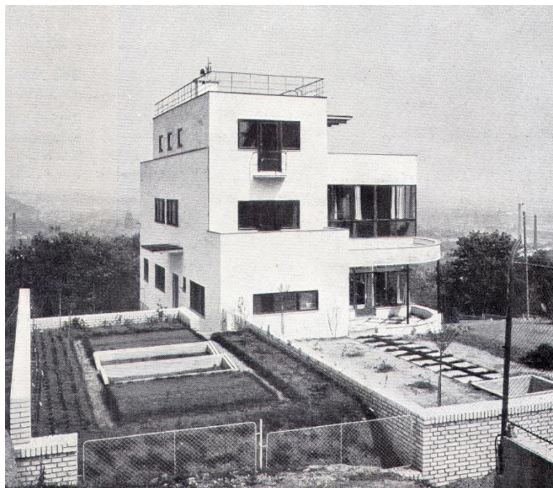
41. J. K. Říha, Vlastní vila se zahradou, Praha-Smíchov, 1929–1930, pohled na užitkovou zahradu a rekreační bazén
