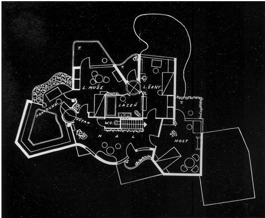
11. Vít Obrtel, Půdorys vily na antický motiv, 1931–1934
