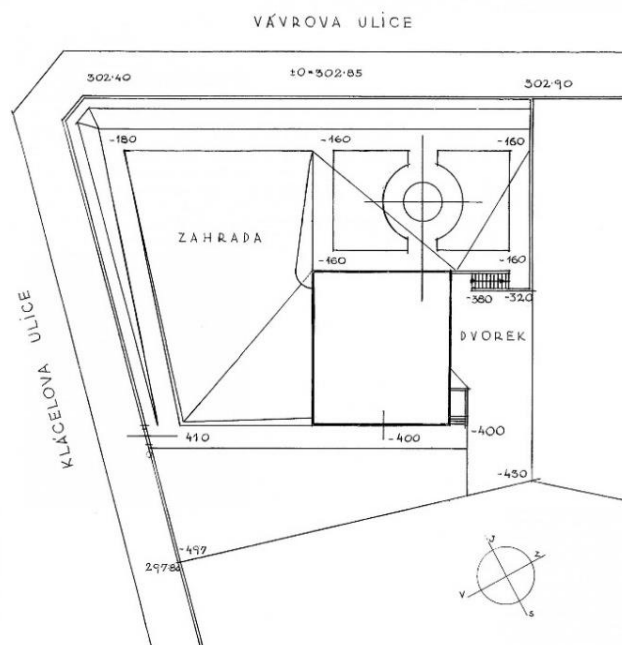
39. Jan Víšek, Situační plán Kudelova domu se zahradou, Brno, 1926–1927
