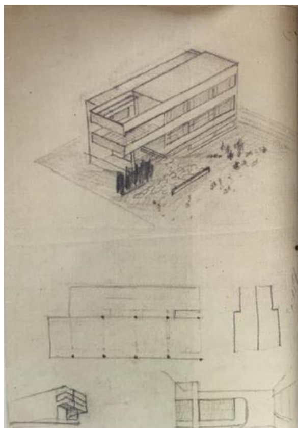
60. Ladislav Žák, Náčrt Zaorálkovy vily se zahradou, nedatováno
