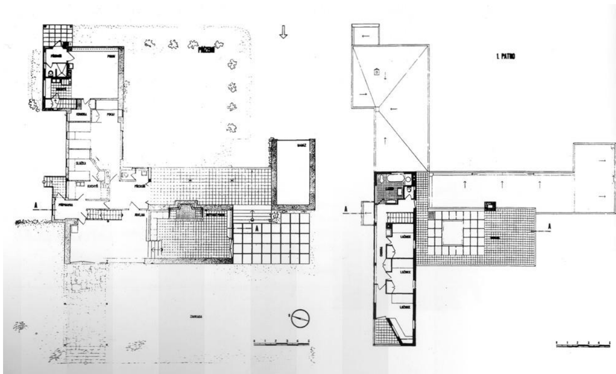
13. Jaroslav Fragner, půdorys Morákovy vily, Nespeky, 1932–1933
