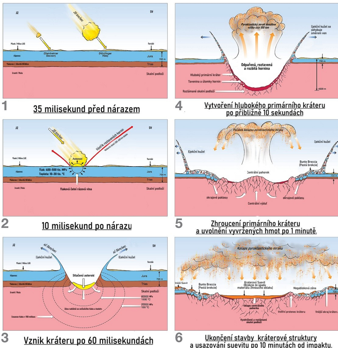
Obrázek 2: Vznik kráteru Ries, dostupné z: https://www.mineralshop.cz/blog-mineralshop/lokality/1283-krater-ries-suevit.html
