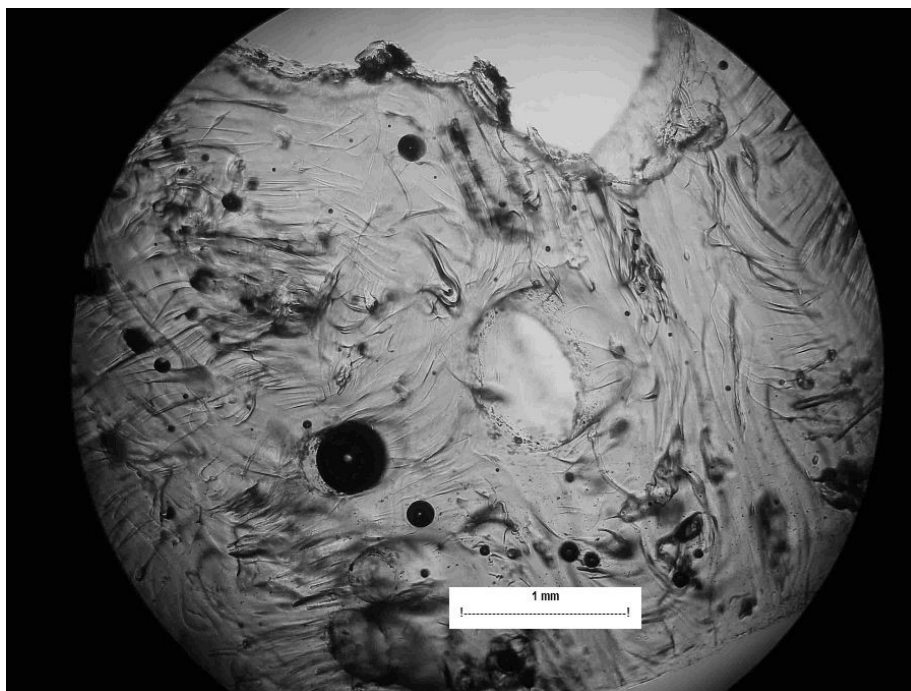
Obrázek 1: Amorfní struktura vltavínu, dostupné z: https://gchmin.ic.cz/casopis/05/05.html
