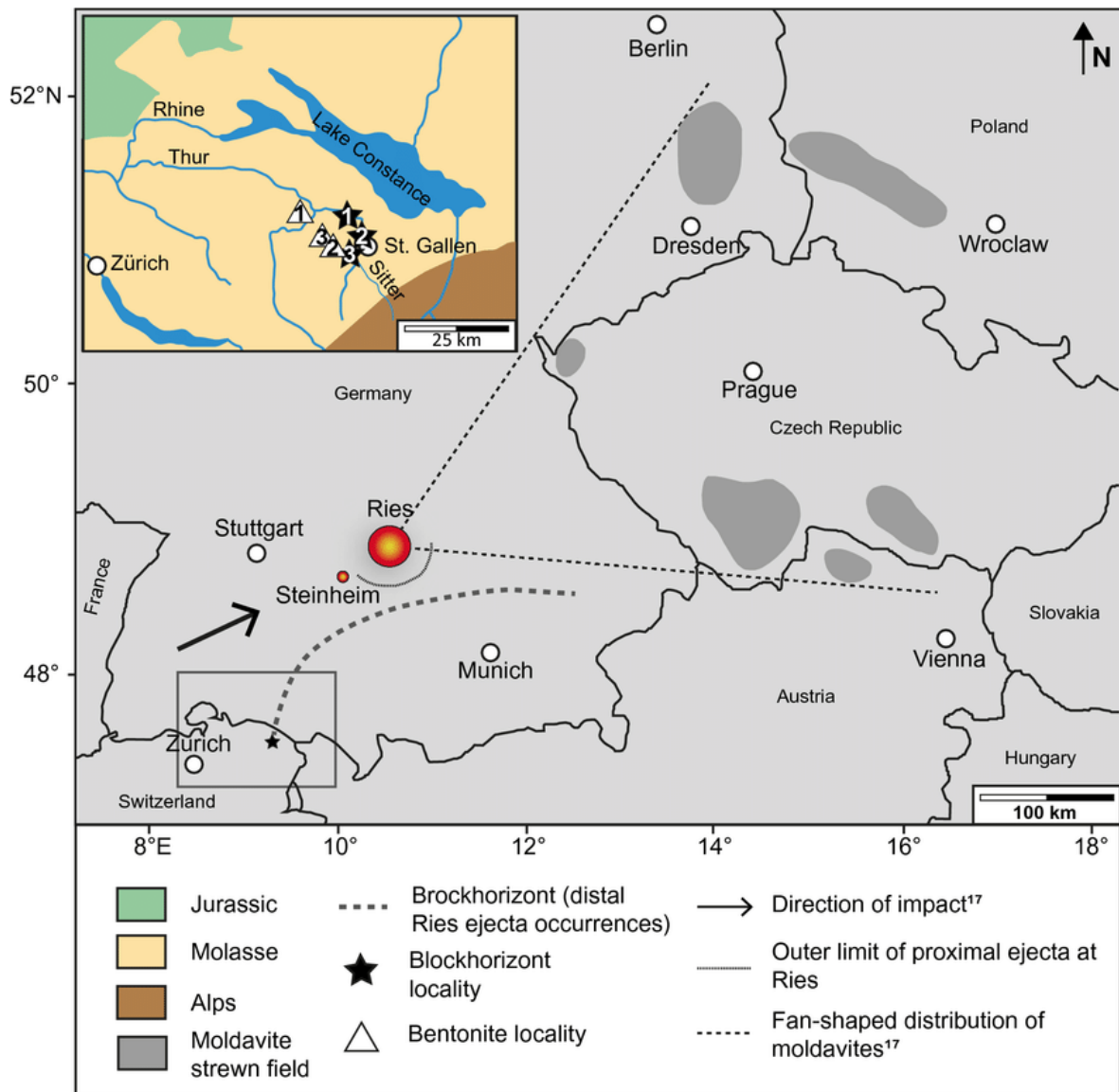
Obrázek 6: Tmavě šedé oblasti náleží vltavínů (nejhojněji však v jižních Čechách a na Moravě). Dostupné z: https://www.researchgate.net/figure/Map-showing-the-location-of-the-Ries-and-Steinheim-impact-structures-along-with-the_fig1_350582581
