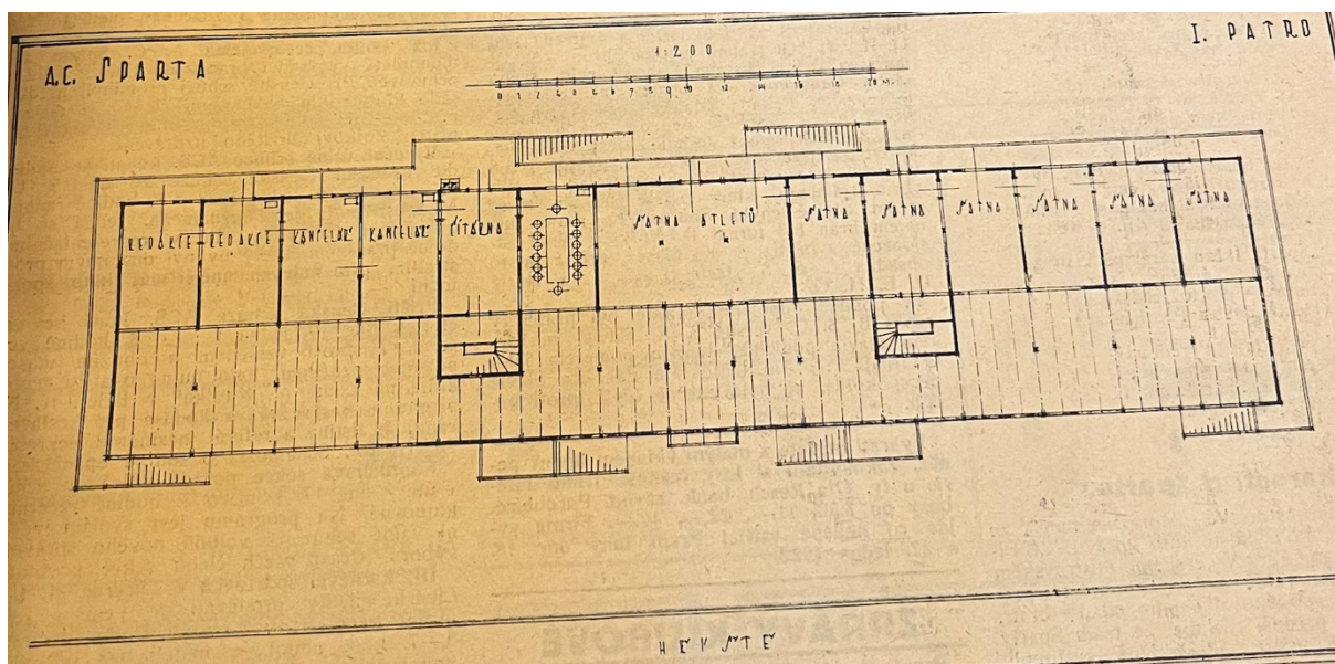
Obr. 5.) Náskres klubovny Sparty (1. patro). Stav z roku 1922.
