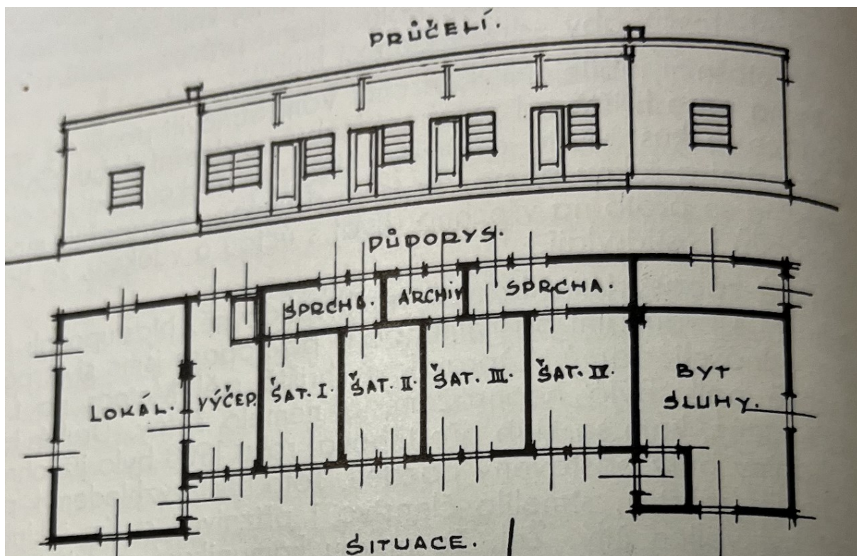
Obr. 4.) Náskres klubovny Meteoru Praha. Stav z let 1934-1936.
