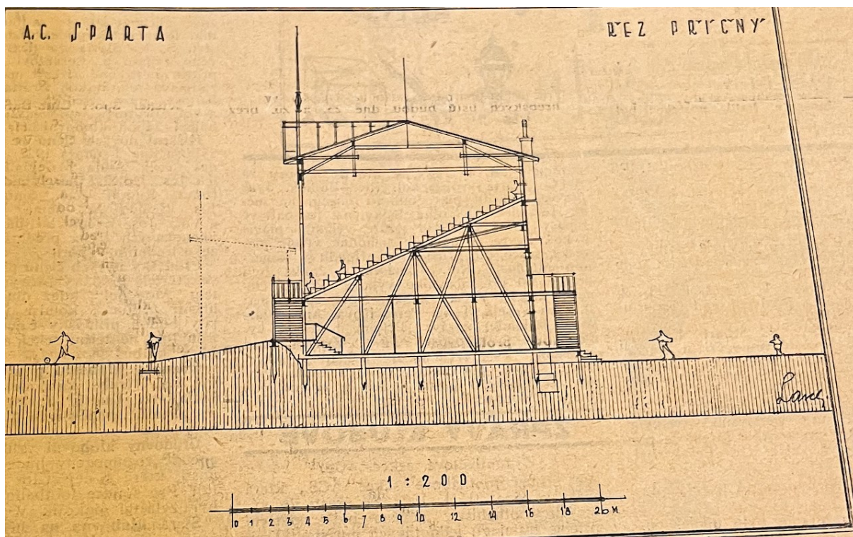
Obr. 6.) Náčres dřevěné tribuny Sparty z roku 1922.
