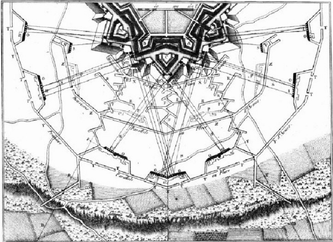
Schéma Vaubanova pravidelného útoku na pevnost. Tři linie paralel, propojené útočnými zákopy – sapami. Racionalizovaně umístěné dělostřelecké baterie cílí na jednotlivé pevnostní prvky. Dole: pevnost Ath, kterou Vauban v roce 1697 během demonstrace svého pravidelného obléhání překvapivě dobyl . Krigsarkivet: 0406:10:008:001 Die Spanische Vestung Ath.
