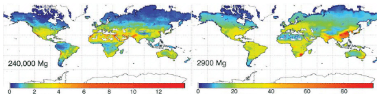
Obr. 5. Model současného uložení emisí Hg uložené v půdách (vlevo, [mg m -2 ]) a půdních emisí Hg (vpravo [μg m -2 rok -1 ]) (Smith-Downey a kol., 2010).
