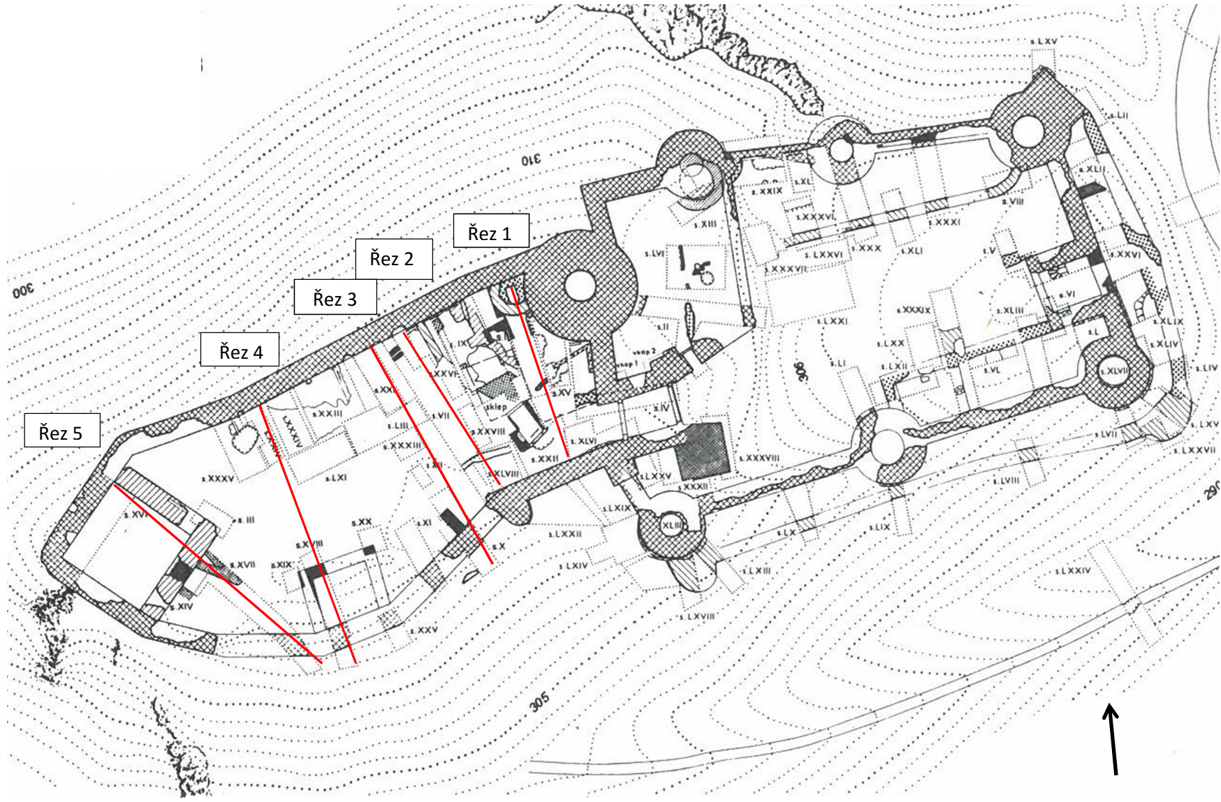
Plán 1: Celkový plán hradu s vyznačením sond (1984), červeně vyznačeny řezy hradem.
