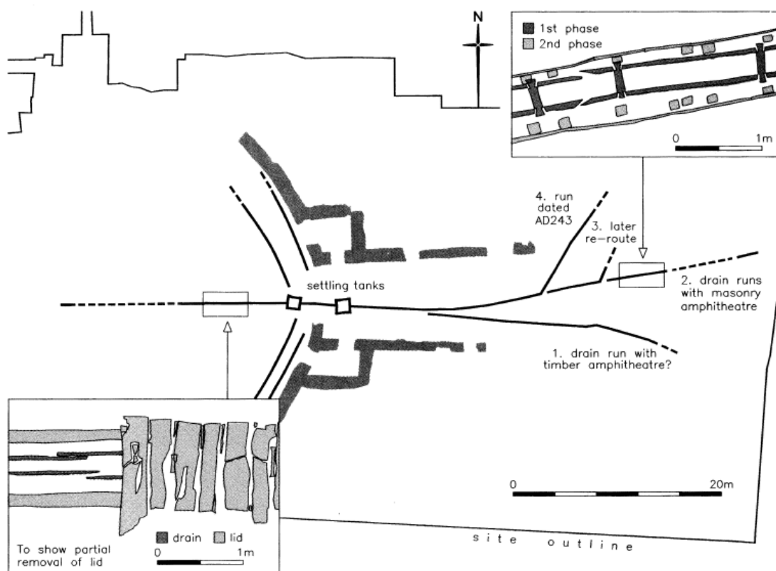
Obrázek 26: Systém odtoku vody z londýnského amfiteátru (Bateman 1997, 60, fig. 40).
