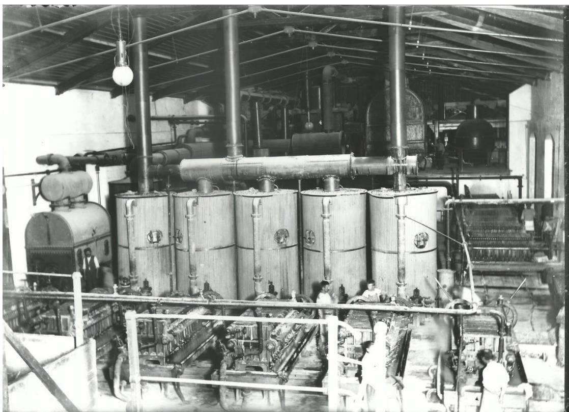
10. Saturační stroje a varna
