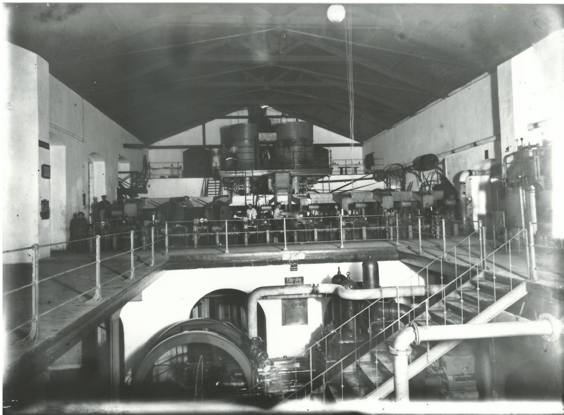
9. Interiér cukrovaru – pohled na řezačky a difuzní stroje
