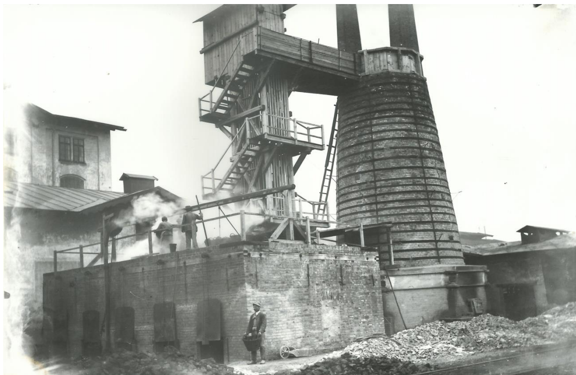
14. Vápenka s hašenkou s komíny v pozadí
