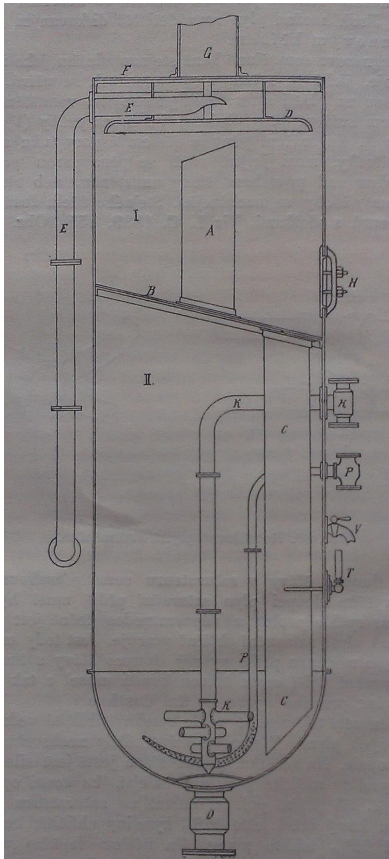
11. Průřez saturačním strojem
